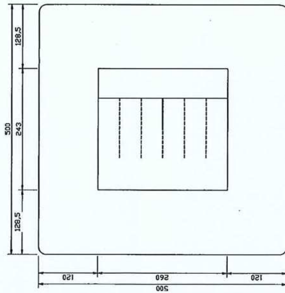
平面図
