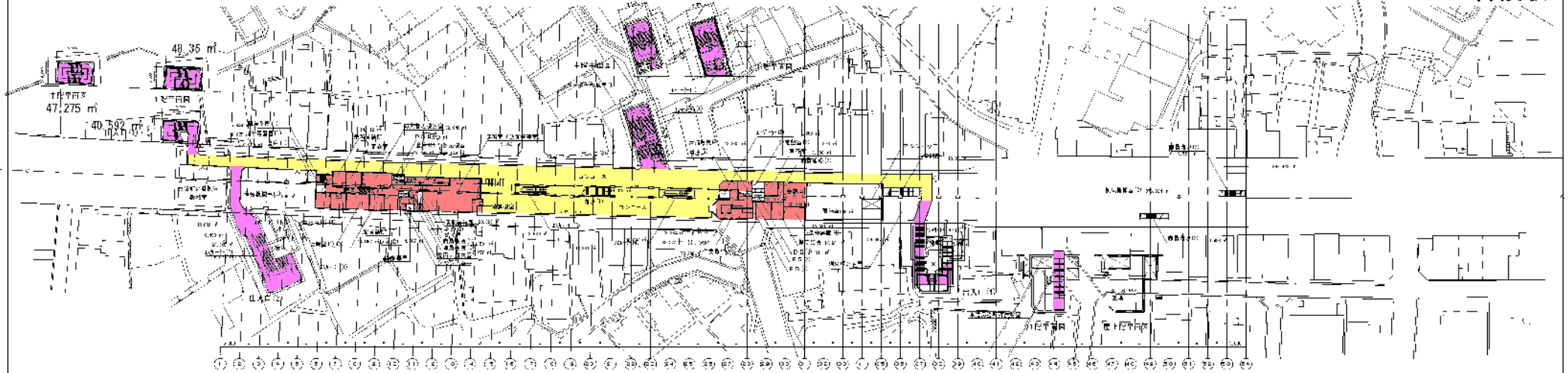
御陵駅 地下1階平面図 S=1/1,000 コンコース階
