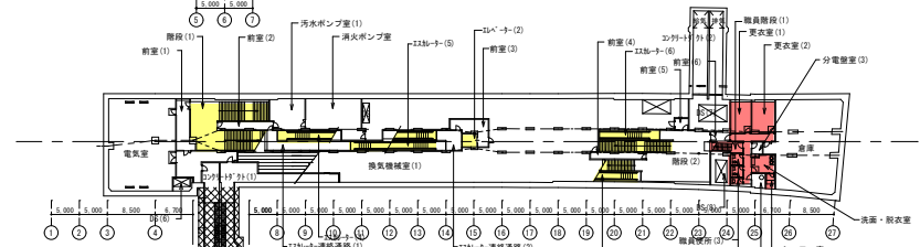
地下2階平面図 中間階
