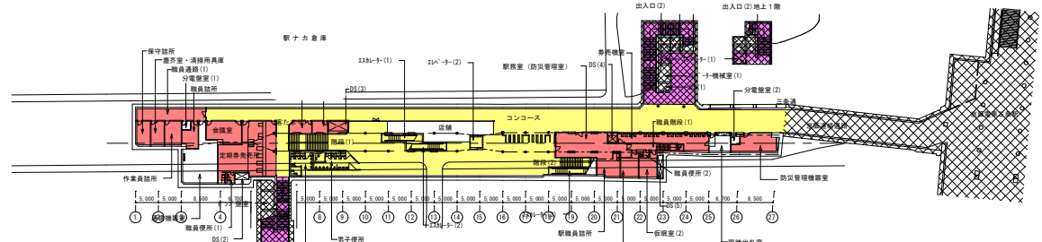
地下1階平面図 コンコース階
