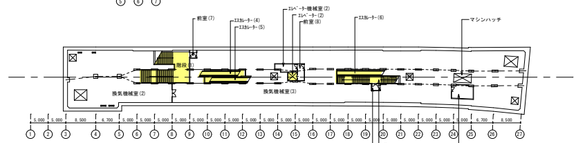
地下3階平面図 中間階
