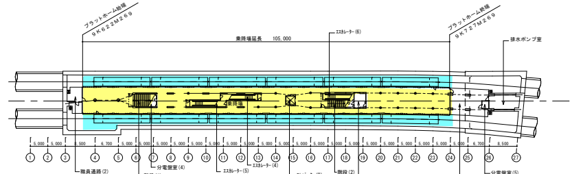
地下4階平面図 ホーム階
