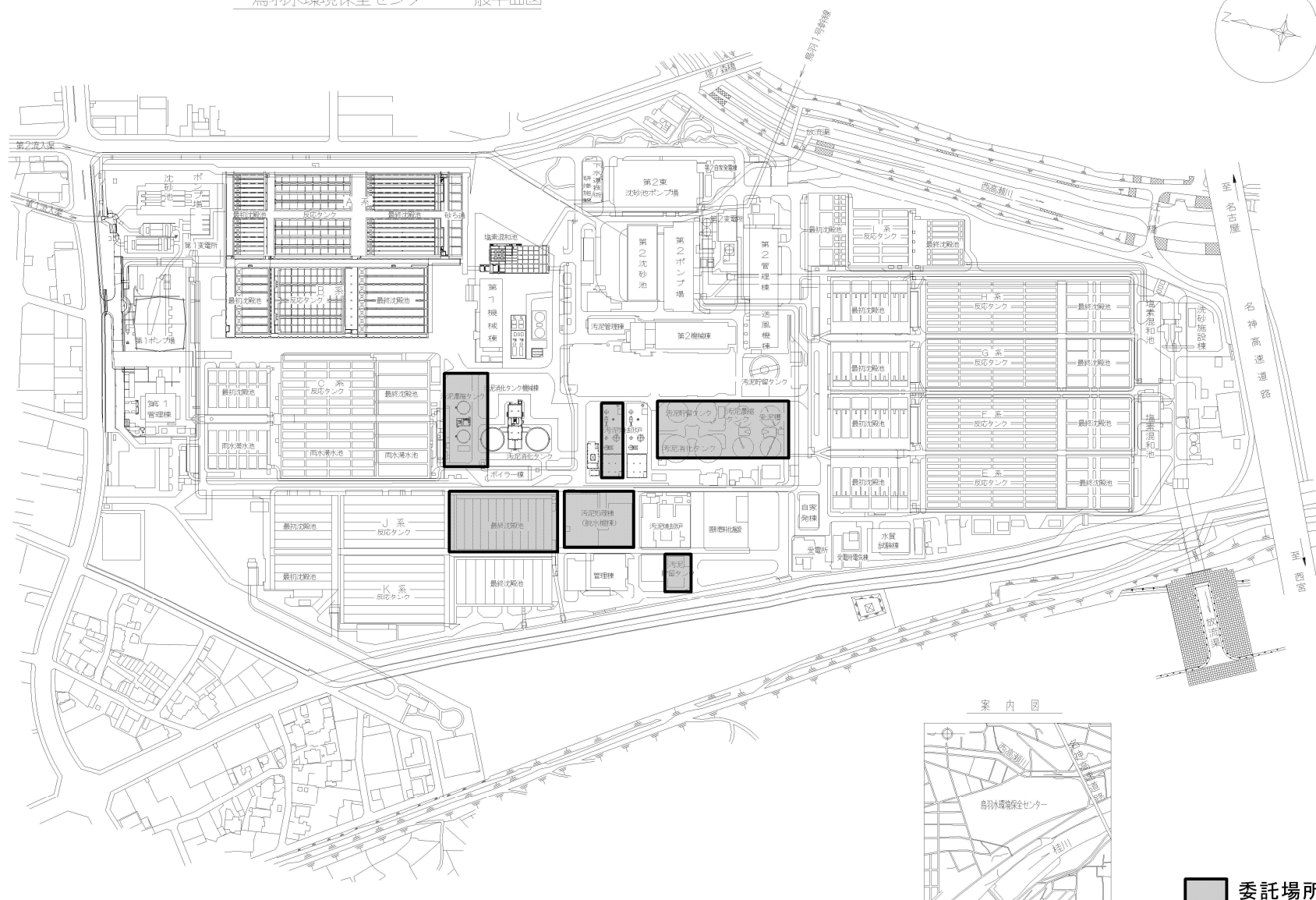
鳥羽水環境保全センター 一般平面図
