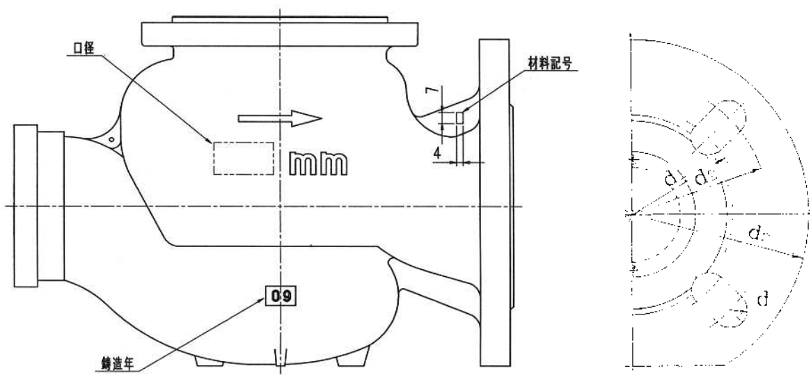
図 1 メーターの外殻図
