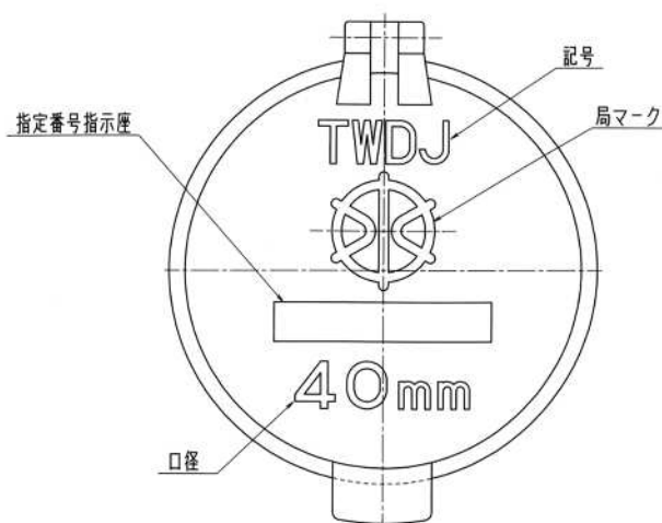
ふた上部
