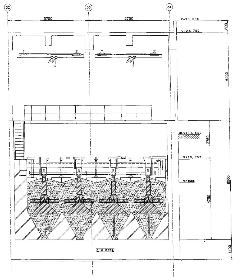
A-A断面図
