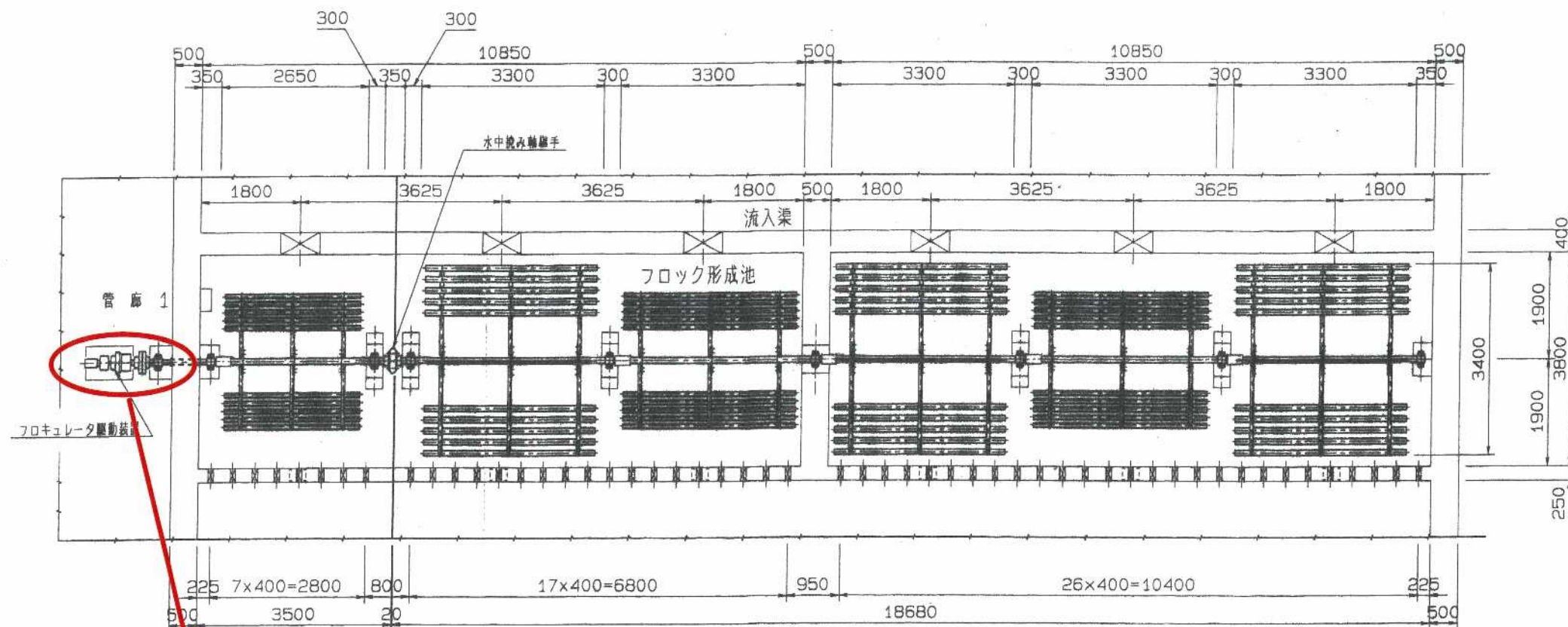
平面図
