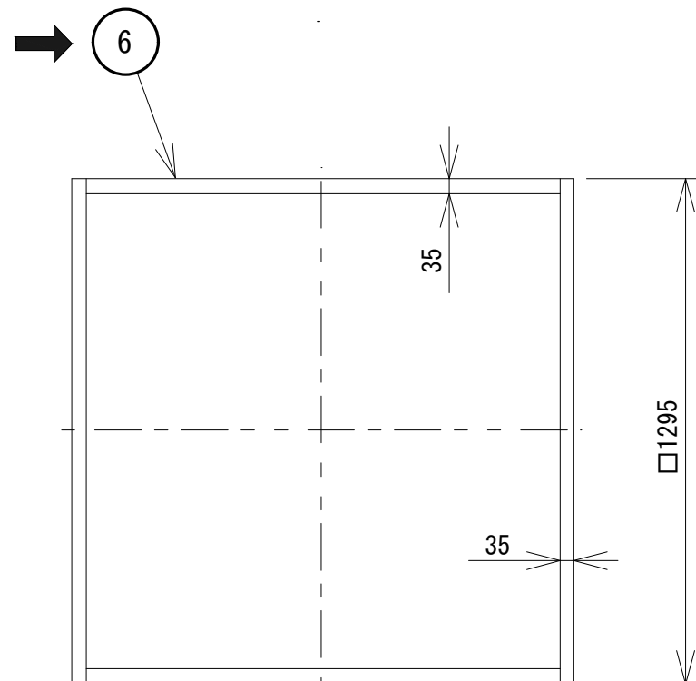
パッキン詳細図
