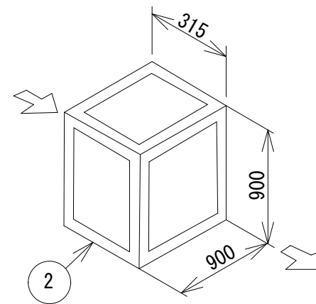
エレメント外形図
