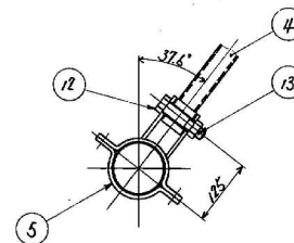
断面 CC (S-XS)
