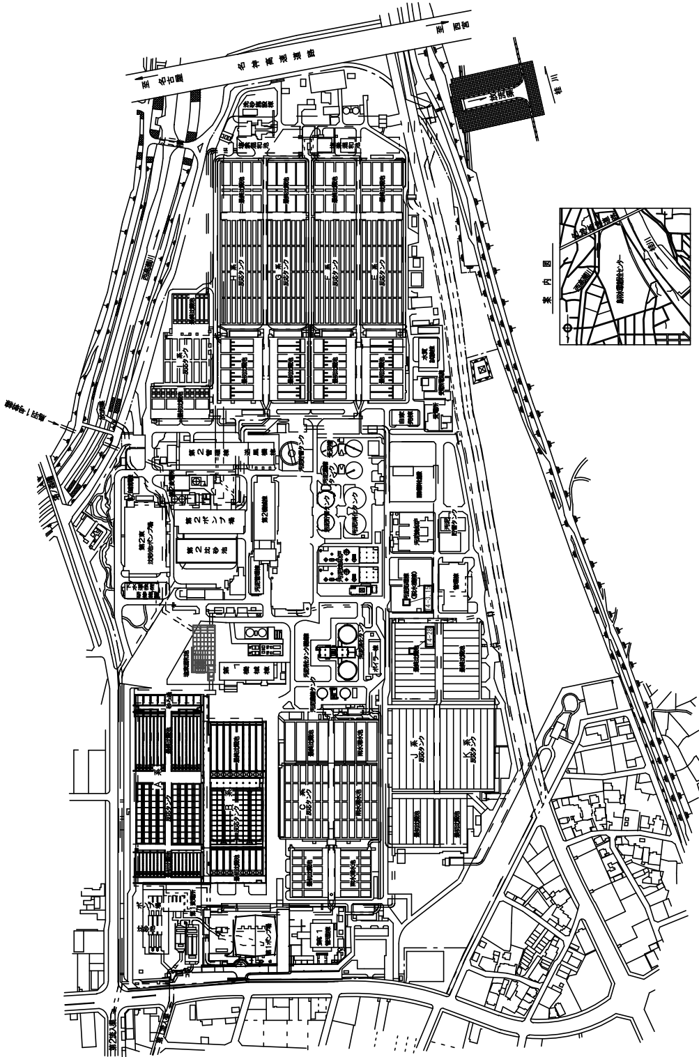
鳥羽水環境保全センター 一般平面図
