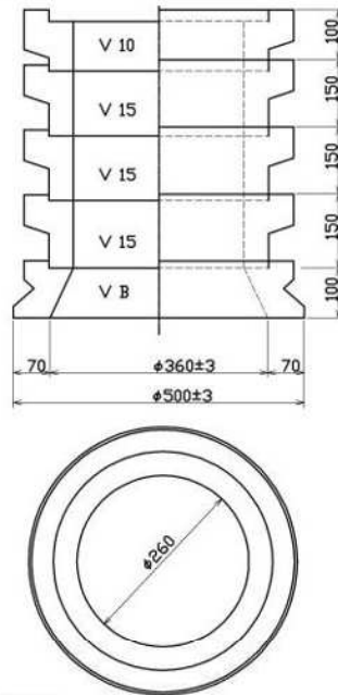
天端調整用
