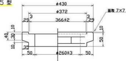
天端調整用
