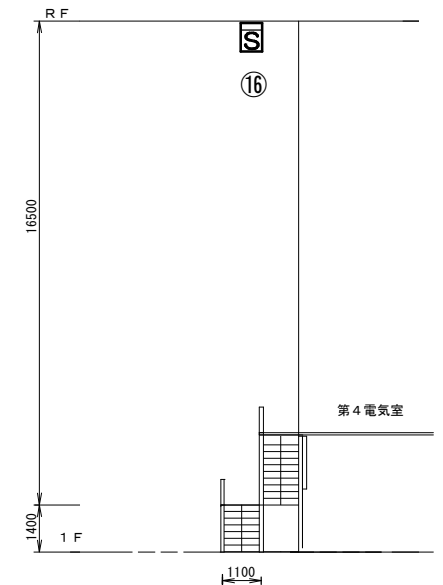
A - A 断面図 (略図)
