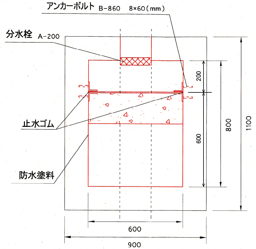
堰板詳細図
