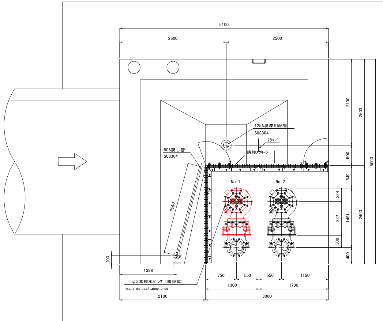
7-7平面矢視図
