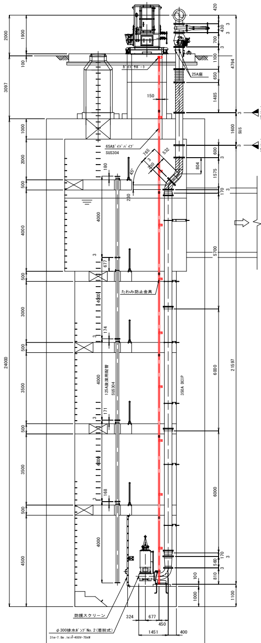
B-B断面図
