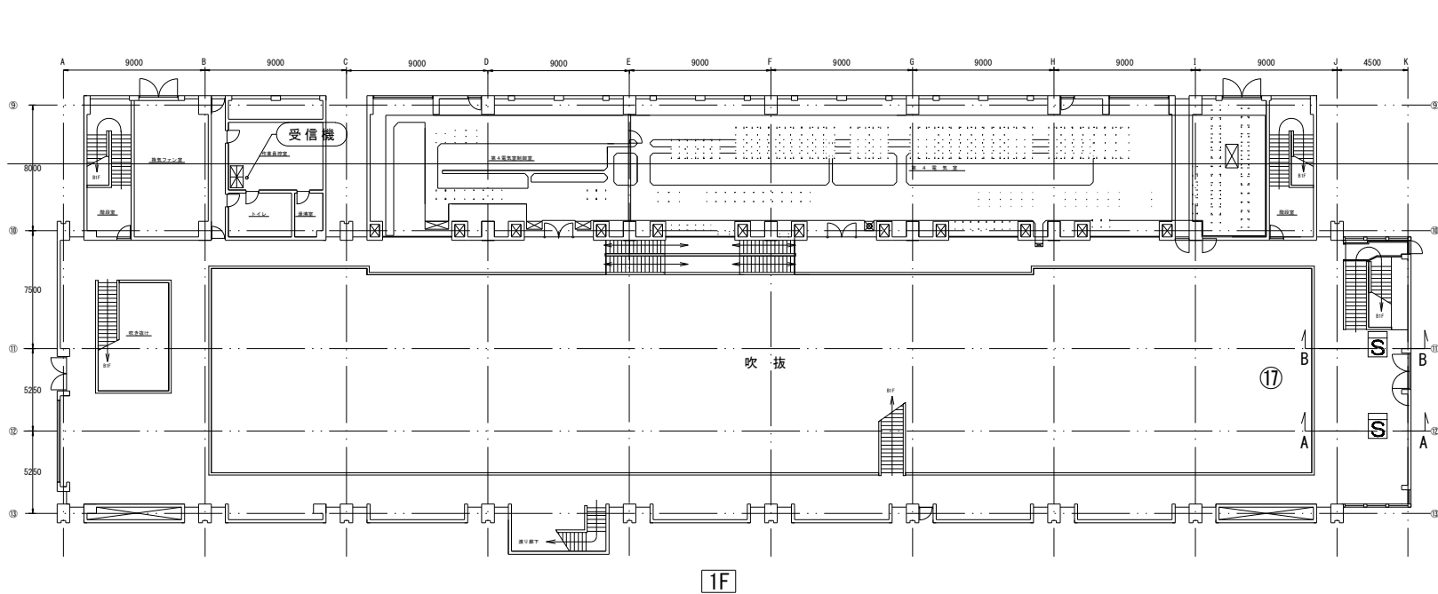
第2ポンプ場 平面図 free
