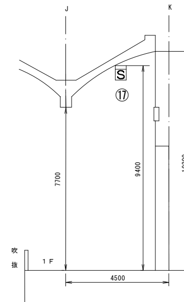
A-A及びB-B断面図（略図）
