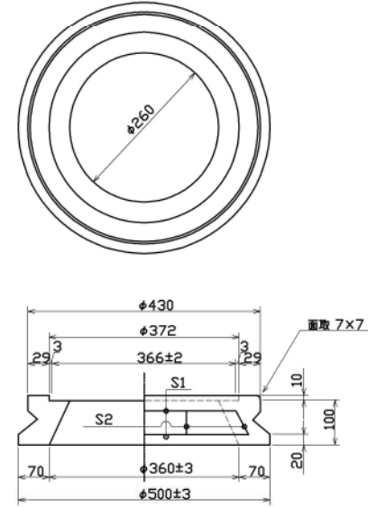
VB 型
