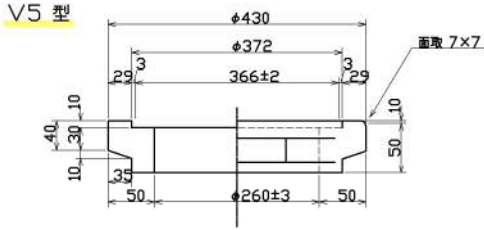
天端調整用
