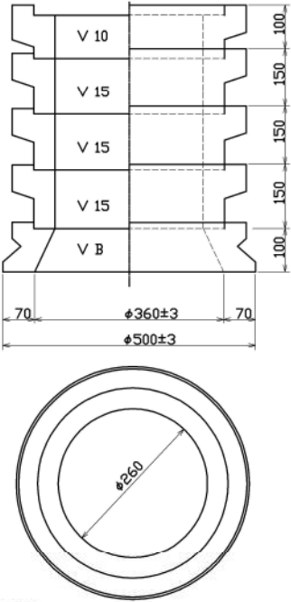
天端調整用
