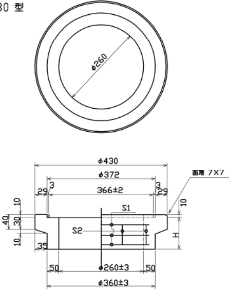
V10.15.30 型
